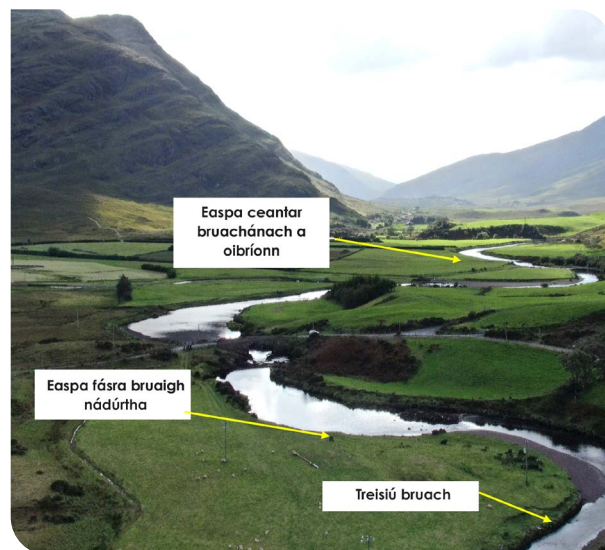
Íomhá: Shamplaí de na hathruithe hidreamoirfeolaíochta is coitianta i ndobharcheantar na hOirimhe.
