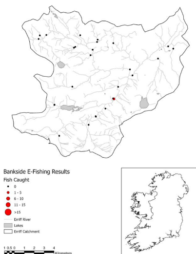
N Torthaí leictriascaireacht cois bhruaigh na hOirimhe 2023
