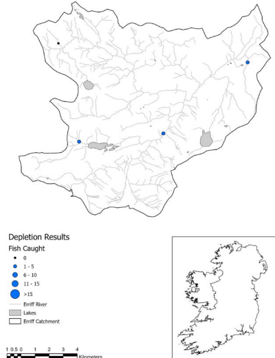
N Torthaí leictriascaireacht ídithe na hOirimhe 2023
