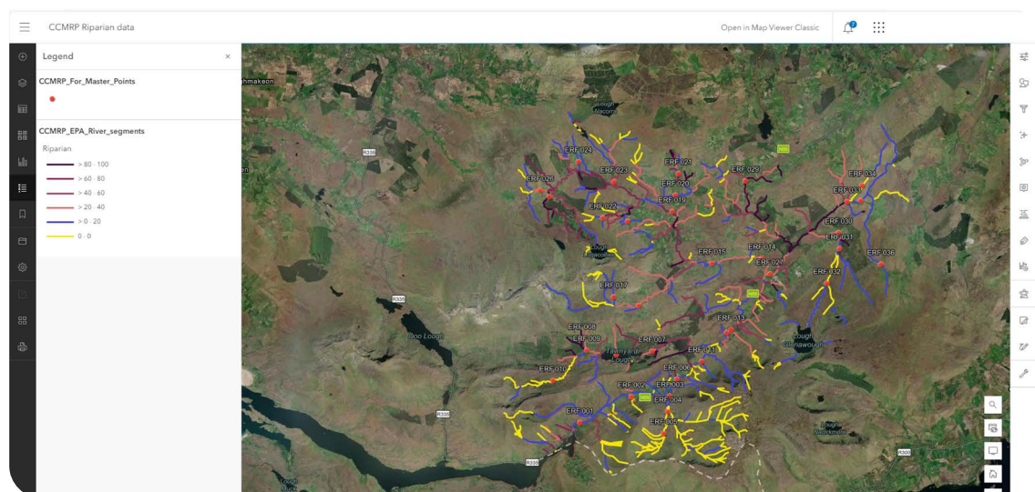
Íomhá: Sampla de mheastacháin ar chlúdach bruachánach i ndobharcheantar na hOirimhe
