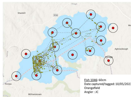
Íomhá: Patrúin ghluaiseachta dhá bhreac gheala ( Salmo trutta ) ar rugadh orthu agus a clibeáladh i Loch Síleann, 2023: a) lasc 1046 (fad: 60 cm) ar rugadh air ar dtús i bPáirc Oráiste agus a braitheadh in áiteanna eile ina dhiaidh sin ar fud an locha. b) lasc 1047 (fad: 38 cm) ar rugadh air ar dtús i gCuan an tSeomraigh an 10/05/2023, ar rugadh arís air an 17/05/2023 agus a braitheadh in áiteanna éagsúla ar fud Loch Síleann é ina dhiaidh sin.
